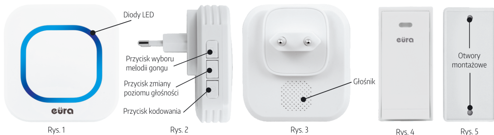
Rys. 1-5. Budowa dzwonka WDP-80H2
