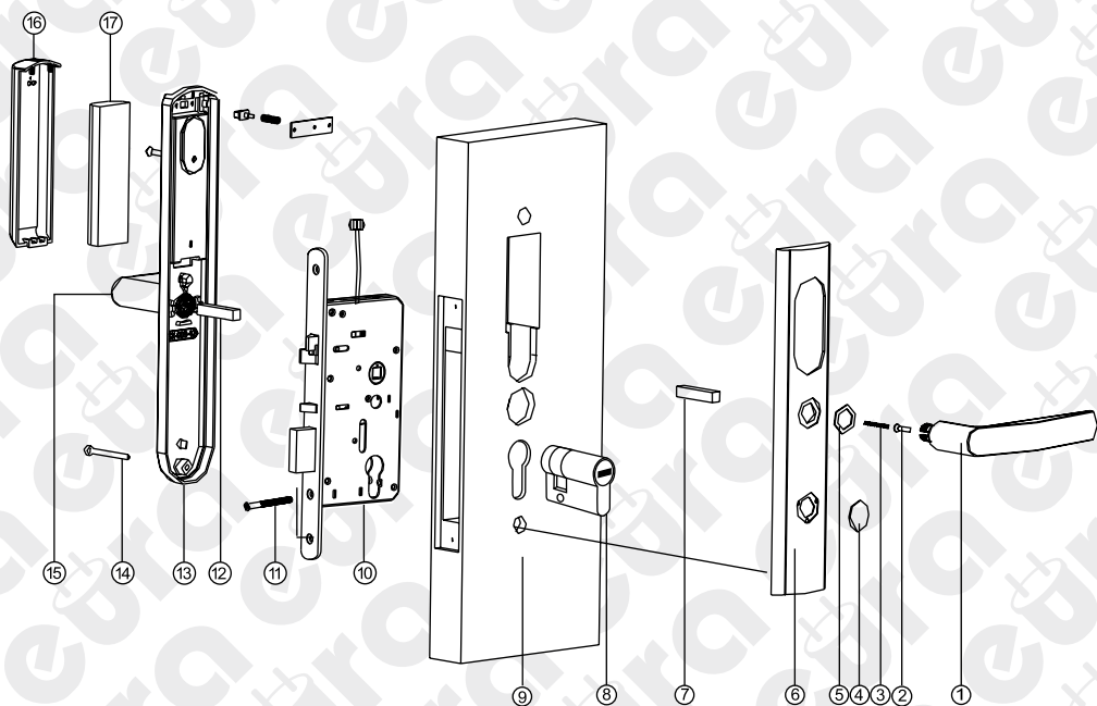
Rys. 3. Budowa kompletnego zamka elektromechanicznego
